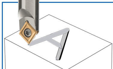
GRAVAGE A 90°
