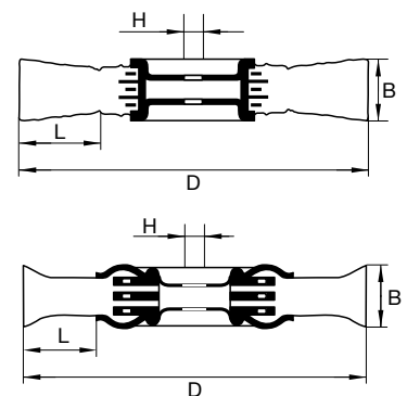
Dimensions brosses circulaires
