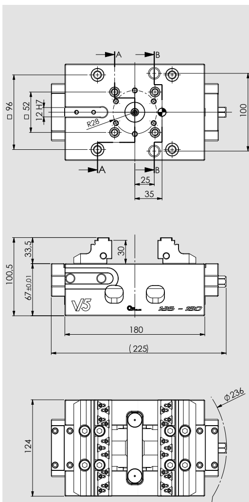
SECTION A-A
