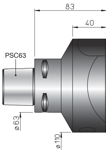
PSC63 - TS80 Ø 120 ~ 200
