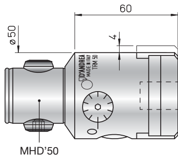
TRM 50 Ø 2.5-108
