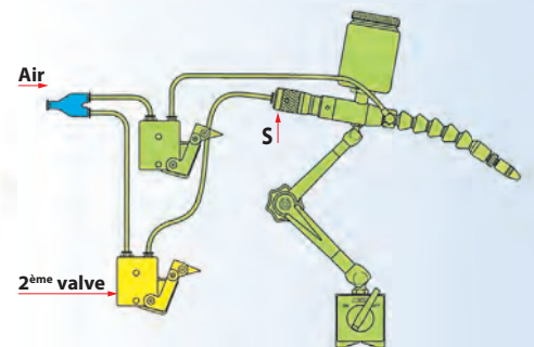
C Montage pour libérer indépendamment goutte à goutte et jet d'air
