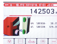
Mesure du diamètre d'un arbre
